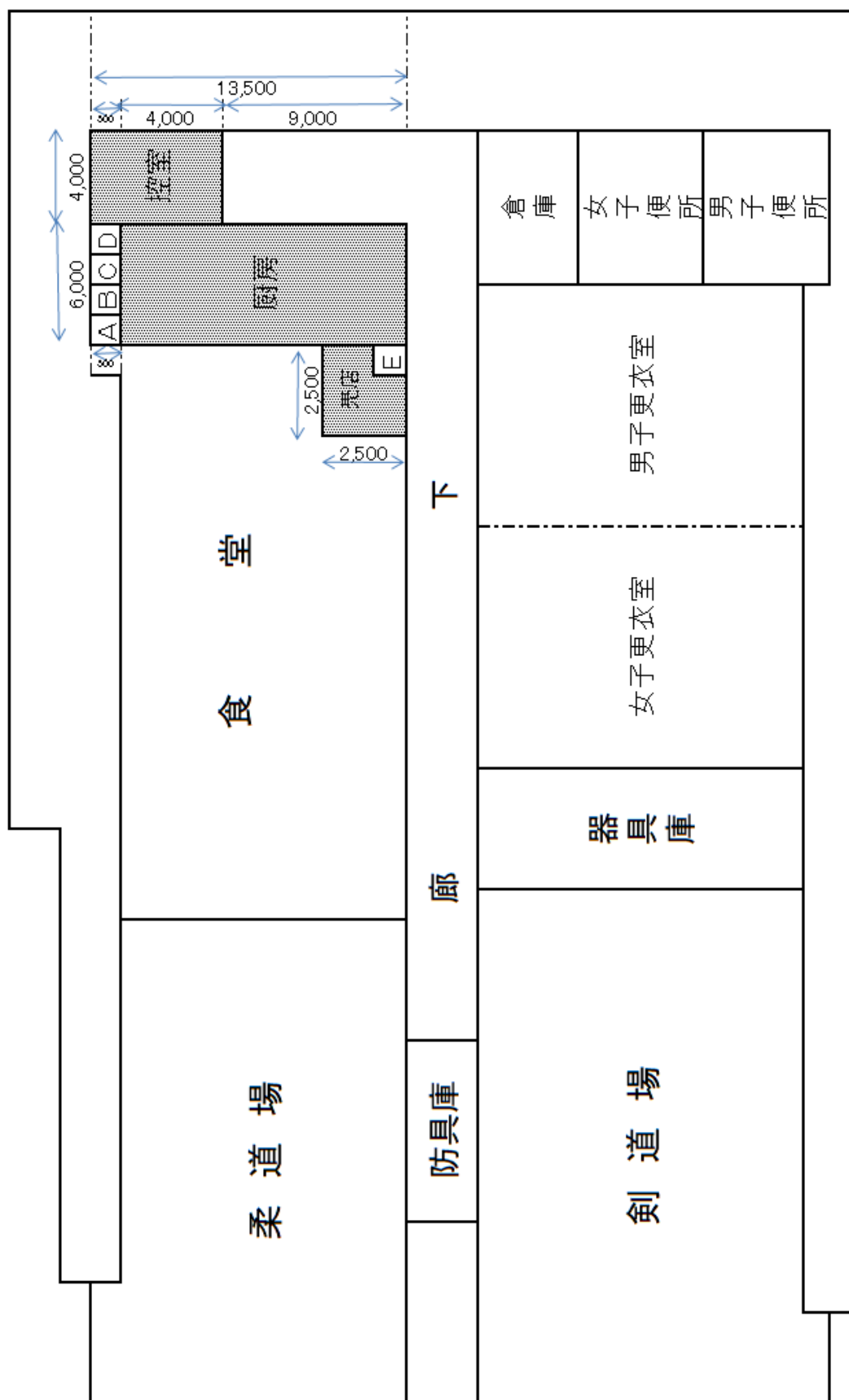
食堂平面图
