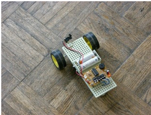
プログラムを組んで台車型ロボットを動かした「自律ロボットの製作実習 2 日目」
