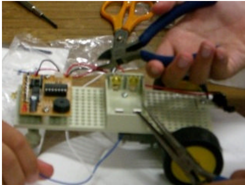
台車型ロボットを製作する「自律ロボットの製作実習 1 日目」
