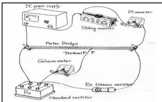
図1 実験装置
