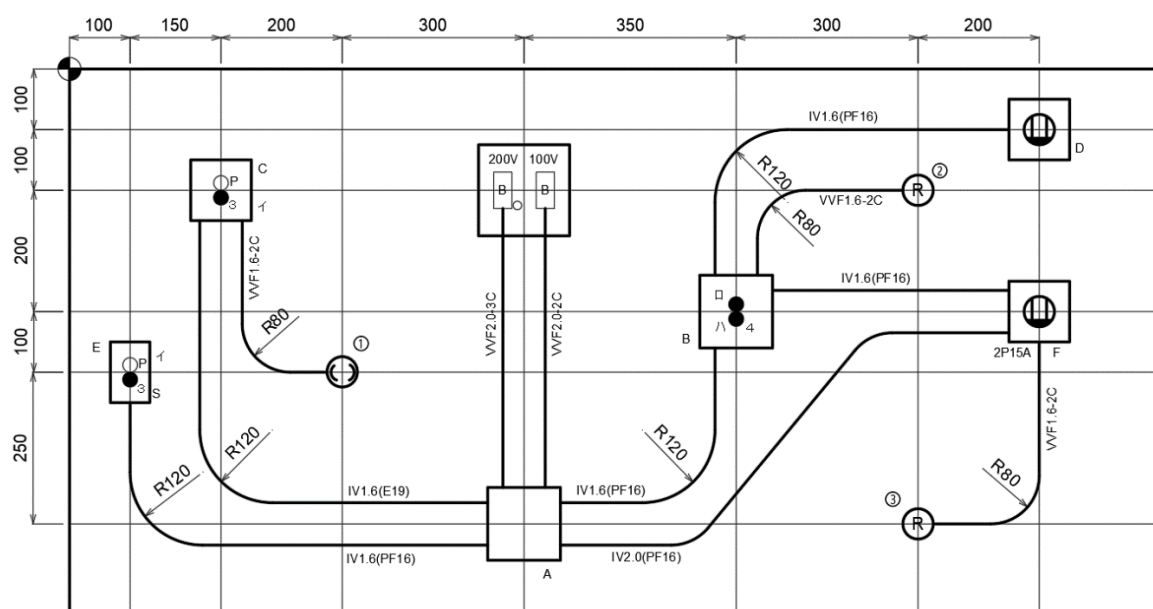
【施工図】
